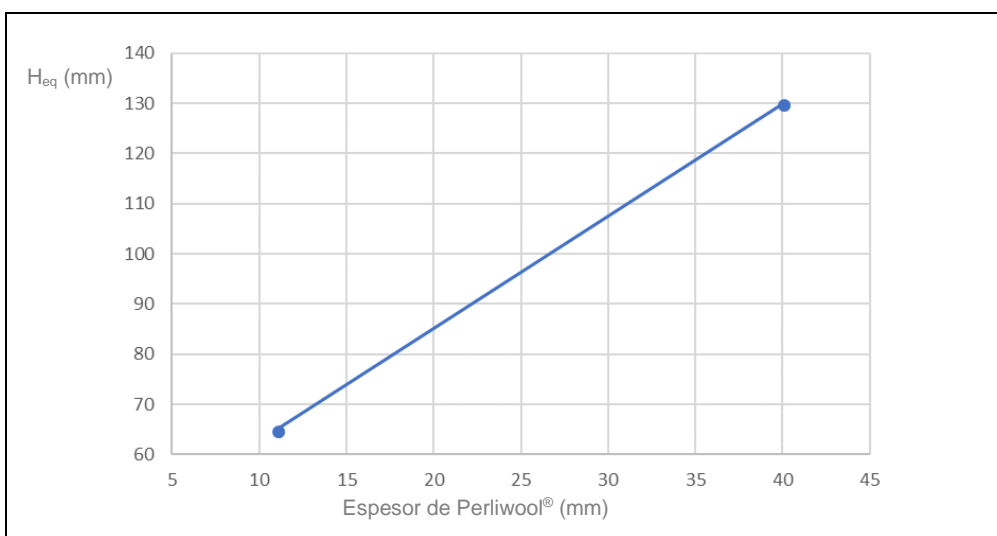
Figura A.2.2.6: Espesor equivalente de hormigón (180 minutos).
